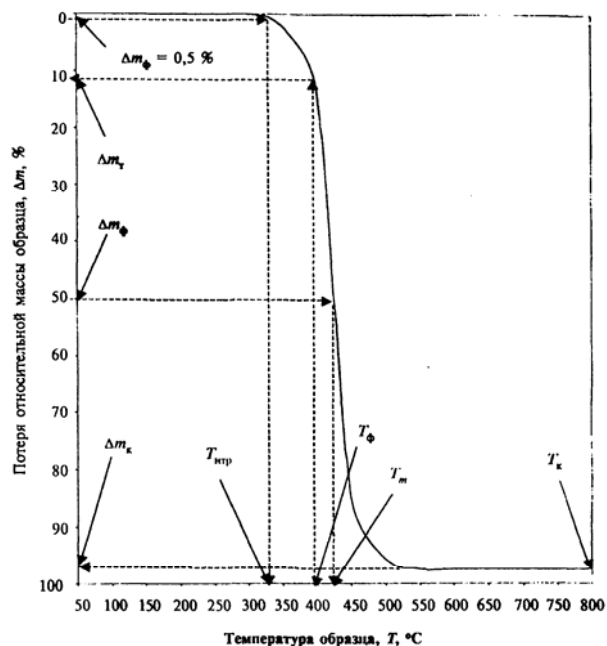
Рисунок А.1 – Пример определения значений потери относительной массы образца по ТГ-зависимости
