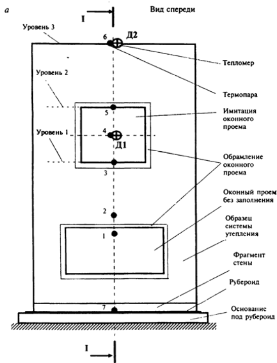
"Рисунок 2а. Схема установки с образцом системы утепления (вид спереди)"
