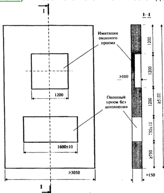
Рисунок 1 — Фрагмент стены
