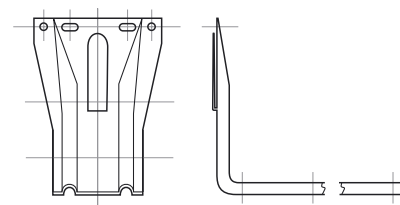
Кронштейн SPIDI max Сталь с алюминиевым покрытием Galvalume Band EN 10215-S250GD+AZ185-A-C DIN 10215
